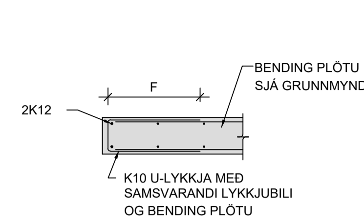
K2 LÓÐRÉTT KENNISNIÐ - PLÖTUBRÚN Mkv. 2
