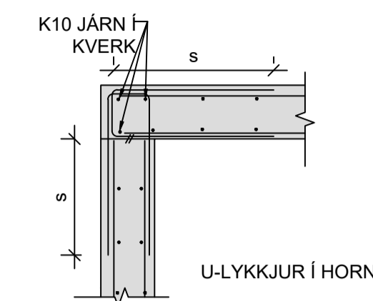
K3 LÁRÉTT KENNISNIÐ - VEGGHORN Mkv. 2
